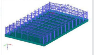
FE-Rechenmodell der Bodenplatte einer Stahlhalle
